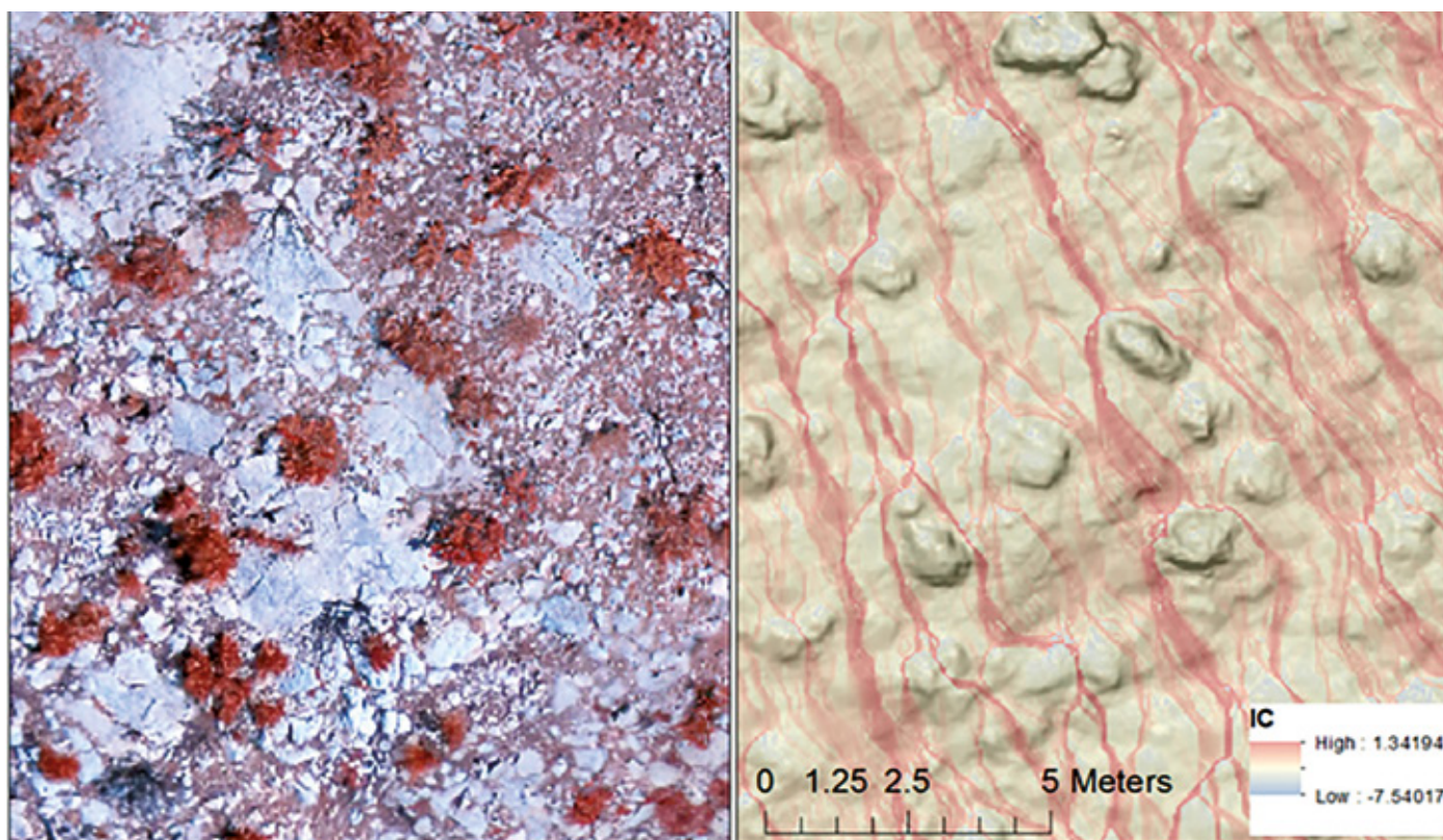
Figura 1. Efectes de la vegetació sobre l'índex de connectivitat dels sediments. La recuperació de la vegetació suposa una disminució de l'índex de connectivitat degut a una major impedància i a provocar un augment de la distància que ha de recórrer cada partícula de sòl fins a la seva deposició. Figura extreta d'Estrany et al., (2015).
