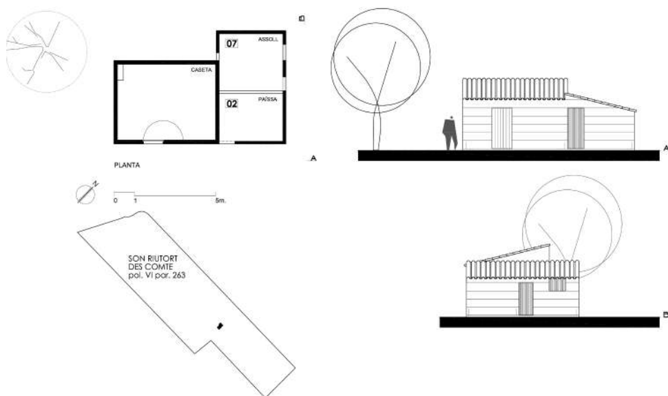
Son Riutort des Comte.
